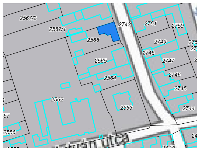
Helyszínrajz
