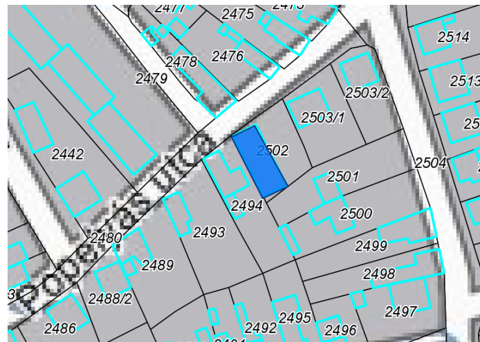
Helyszínrajz
