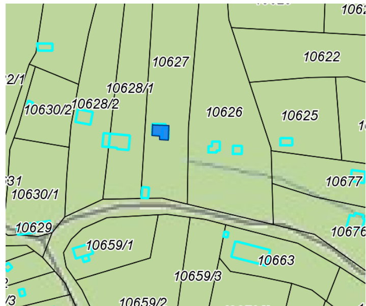
Helyszínrajz
